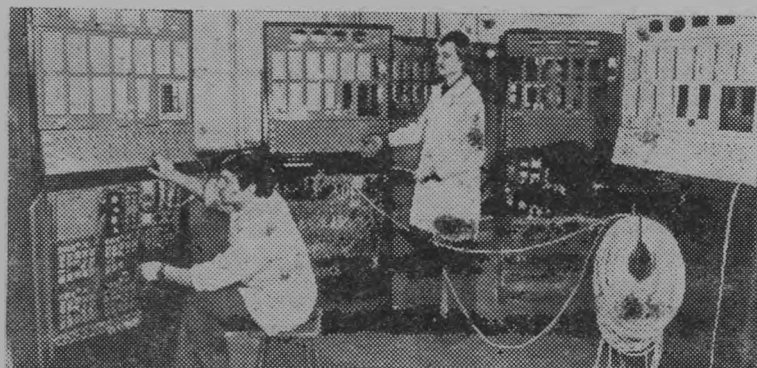
Казахская ССР. С конвейера Усть-Каменогорского завода приборь сошли первые пневматические управляющие машины — «ПУМ-1А», предназначенные для автоматизации процесса гранулирования кормов в животноводстве.
