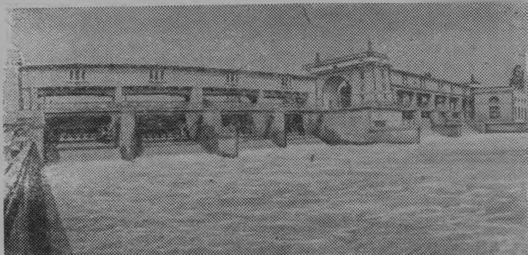
Северо-Осетинская АССР. Живительной артерией плодородия, напоившей сотни тысяч гектаров полей и садов хозяйств Северного Кавказа, стал Терско-Кумский канал.
