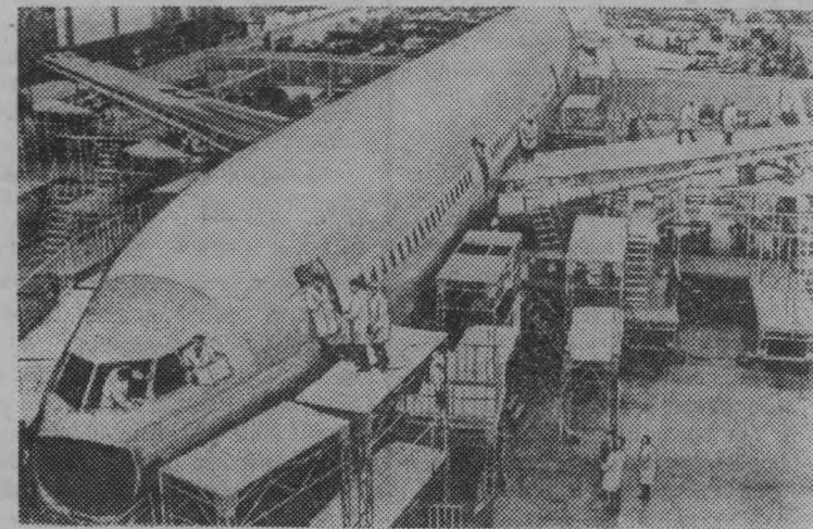
Работники Воронежского ордена Ленина авиационного завода, претворяя в жизнь решения XXV съезда КПСС, осваивают производство широкофюзеляжных самолетов ИЛ-86. Такой самолет сможет взять на борт 350 пассажиров. Оптимальная крейсерская скорость машины 900—950 км/час, высота полета 9—10 тысяч метров.
