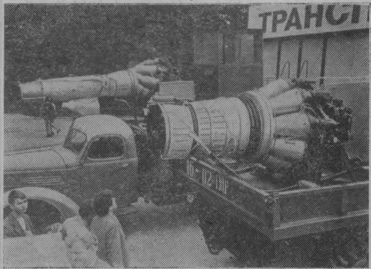
Москва. Авиадвигатели, отработавшие свой срок в воздухе, можно широко использовать в народном хозяйстве. Об этом рассказывает тематическая выставка «Наземное применение авиадвигателей в народном хозяйстве, открытая на ВДНХ СССР».
