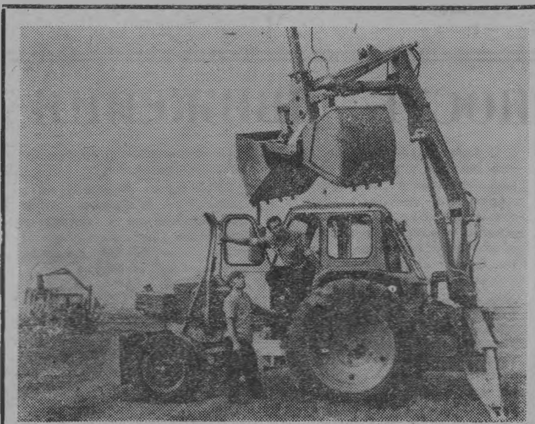
Ивано-Франковская область. На заводе «Коломысельмаш» ведется подготовка к производству нового погрузчика-экскаватора ПЭ-0,8 Б. В новой модели улучшена система управления, усилена конструкция бульдозера, упрощены возможности переоборудования машины из погрузчика в экскаватор. Погрузчик снабжен ковшем для сыпучих грузов, когтями для соломы и навоза, экскаваторной лопатой для рытья траншей, крюком для упакованных грузов. Грузоподъемность машины — 800 килограммов. На снимке: во время испытания погрузчика-экскаватора ПЭ-0,8 Б. Фото В. Миговича. (Фотохроника ТАСС).
