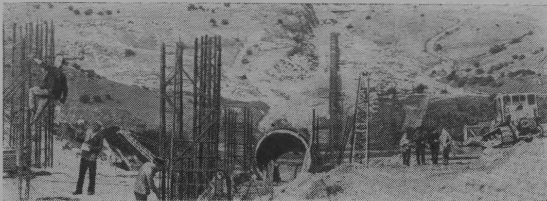
Ставропольский край. В сложных топографических условиях пересеченной местности прокладывается русло третьей очереди Большого Ставропольского канала. Гидростроителям предстоит смонтировать три металлических дюкера и проложить семикилометровый тоннель.
