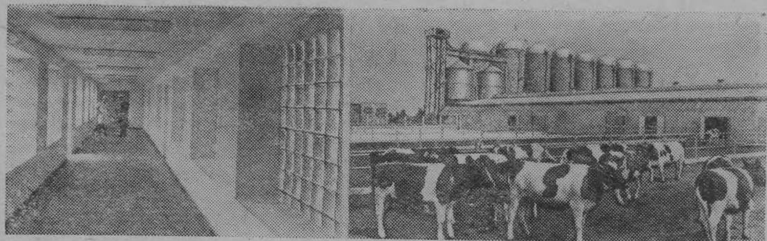
Московская область. В нескольких километрах от города Подольска вырос новый молочно-промышленный комплекс «Щапэво», оборудование которого поставлено из ГДР. Пока он единственный в стране. В нем разместится 2000 коров, которых будут обслуживать операторы машинного доения и операторы по раздаче кормов. Инженеры и техники будут поддерживать необходимый режим этого сложного автоматизированного животноводческого хозяйства, стоя у
