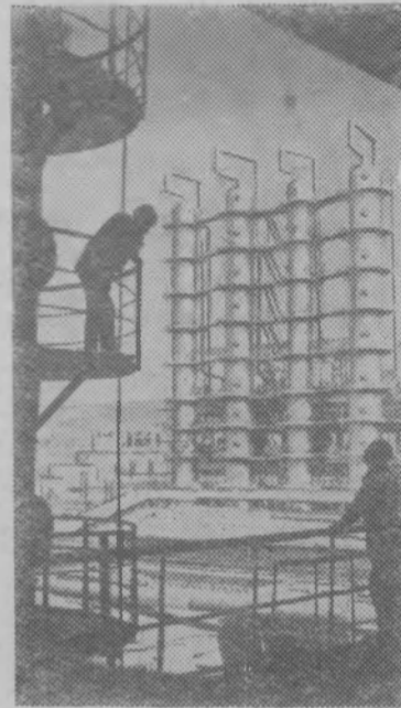
Ереван. Отделение ректификации завода «Поливинилцелат».
