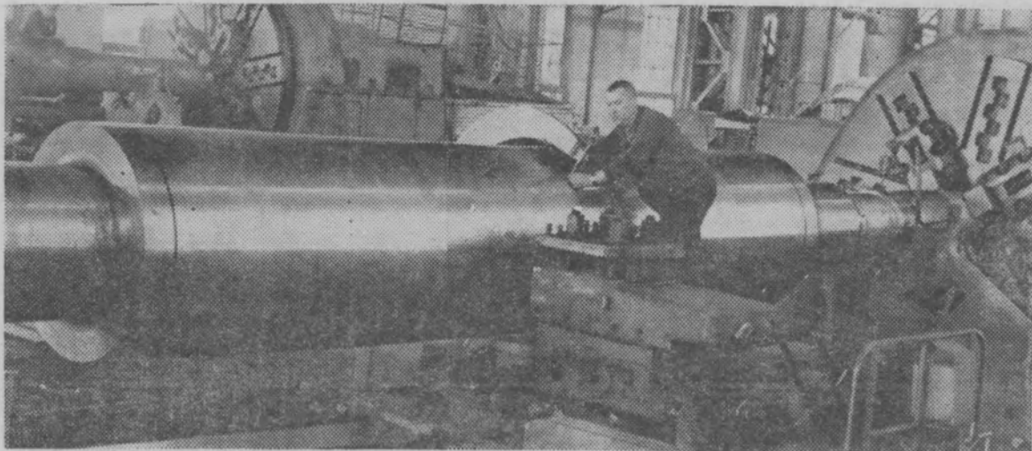
Украинская ССР. На харьковском заводе «Электротяжмаш» имени В. И. Ленина идет изготовление крупнейшего в мире однофазного турбогенератора мощностью 500 тысяч киловатт.
