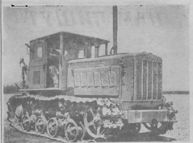
Азербайджанская ССР. На Закавказской машиноиспытательной станции проходит испытания новый трактор «Т-74». Он предназначен для работы с прицепными и навесными орудиями на повышенных скоростях до 10,2 километра в час. Новая машина по сравнению с серийным образцом трактора этого типа «ДТ-53» имеет целый ряд преимуществ. На нем установлен более мощный мотор «СМД-14А» завода «Серп и молот» с некоторым снижением расхода топлива. Запуск двигателя производится электростартером. В кабине водителя имеются вентилятор и обогревательное устройство.
