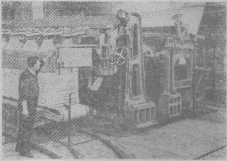
ПЕРМСКАЯ ОБЛАСТЬ. На Соликамском целлюлозно-бумажном комбинате механизирован процесс резки, транспортировки и упаковки целлюлозы, поступающей от прессы. На снимке: общий вид самоклада прессы. Фото Е. Загуляева. Фотохроника ТАСС.
