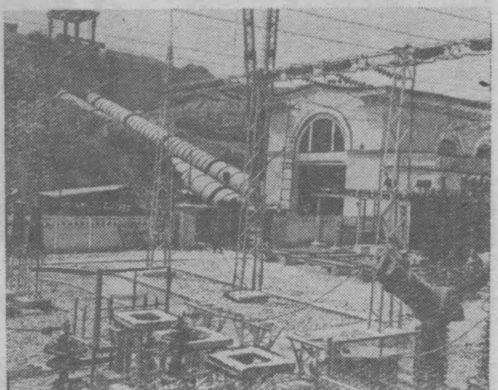
Дагестанская АССР. На реке Сулак заканчивается сооружение крупнейшей на Северном Кавказе Чирюртовской ГЭС. Сейчас ведется наладка оборудования.
