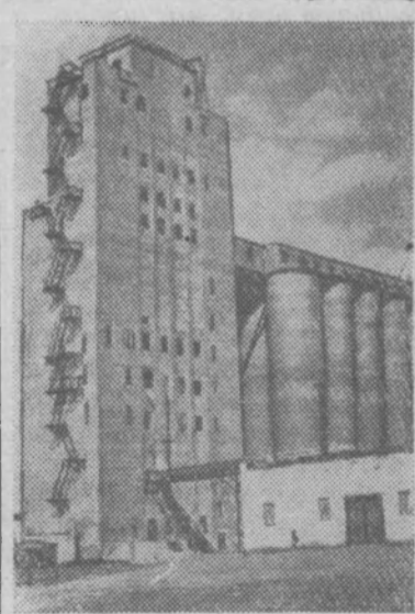
КУРГАНСКАЯ ОБЛАСТЬ. В Далматове закончено строительство первой очереди элеватора емкостью 13 тысяч тонн зерна. Он будет принимать хлеб непосредственно от комбайнов, с любой влажностью. Для контроля работы механизмов установлен щит управления. Диспетчер будет отдавать команды по микрофону. Обслуживающий персонал будет подниматься в верхние этажи на лифте. На снимке: новый элеватор в Далматове. Фото С. Юдина. Фотохроника ТАСС.
