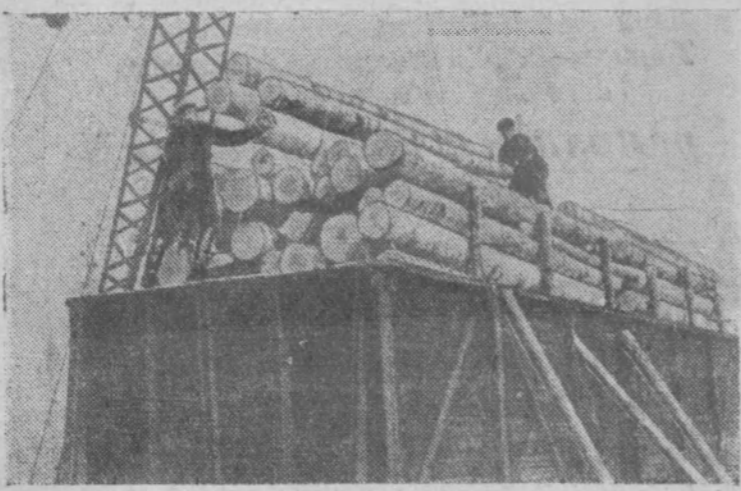
Такой лес отправляют пижемские лесозаготовители новостройкам нашей Родины. На снимке: погрузка леса в вагоны широкой колеи прогрессивным методом «шапкой».
