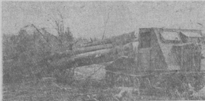
Майский лесоучасток. На снимке: трелевка леса с кронами.
