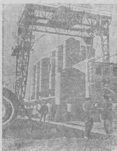
Азербайджанская ССР. В Кировабаде сооружается крупный глиноземный завод. В этом году будет закончено строительство сернокислотного цеха с металлическими емкостями высотой 20—25 метров. На снимке: строительство сернокислотного цеха глиноземного завода. Фото О. Казиева.
